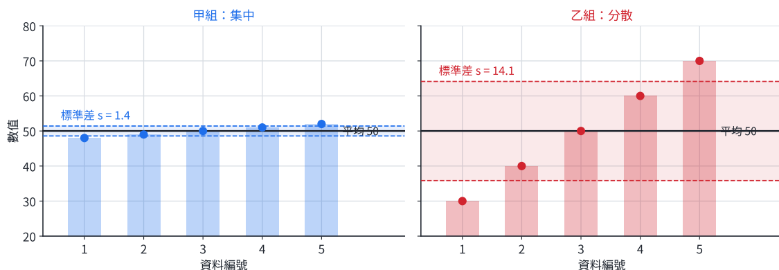
圖 4-1：兩組資料平均數都是 50，但甲組擠在平均附近（標準差約 1.4），乙組散得很開（標準差約 14.1）。標準差越大，資料越分散。
