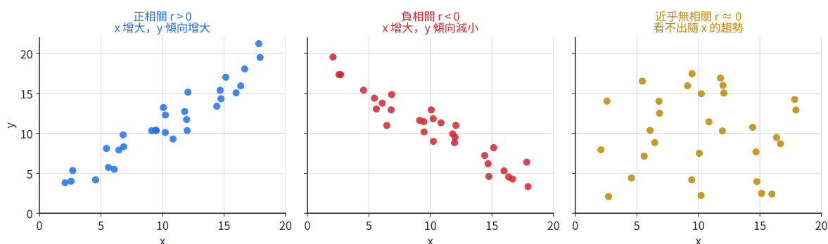
圖 4-3：散布圖的三種走向。左——正相關（左下到右上）；中——負相關（左上到右下）；右——近乎無相關（看不出隨 x 的趨勢）。
