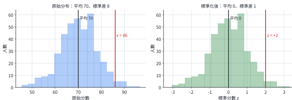
圖 4-2：原始分布平均 70、標準差 8，原始分數 86 在平均上方 2 個標準差處；標準化後整個分布平移縮放，原來的 86 對應到 z = +2 。
