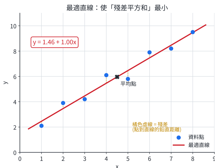
圖 4-4：橘色虛線是各點的殘差（資料點到直線的鉛直距離）。最適直線就是讓這些殘差「平方後加起來」最小的那條，且必通過平均點。
